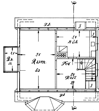
Vindsplan.
