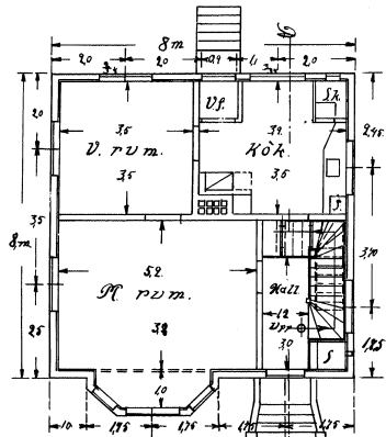
Boiten plan.
